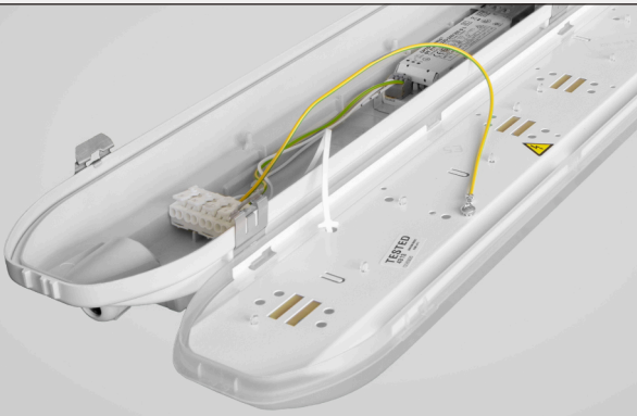
Ventilační ucpávka
