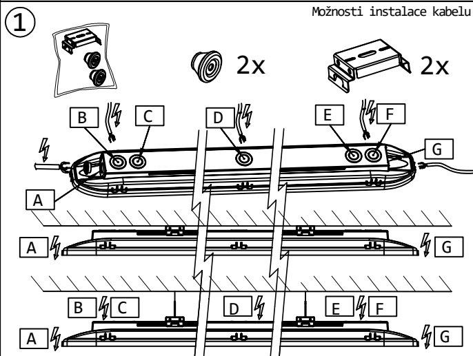
Možnosti instalace kabelu
